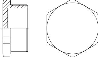
Метрическая резьба, трубная цилиндрическая резьба
